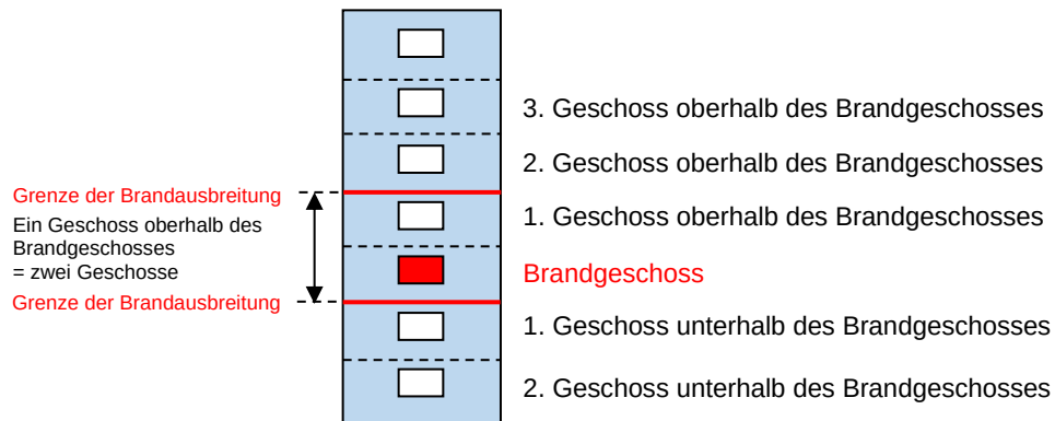
Abbildung 1: Darstellung des Schutzziels für Fassaden nach (OIB) – «zwei Geschosse» [4]
