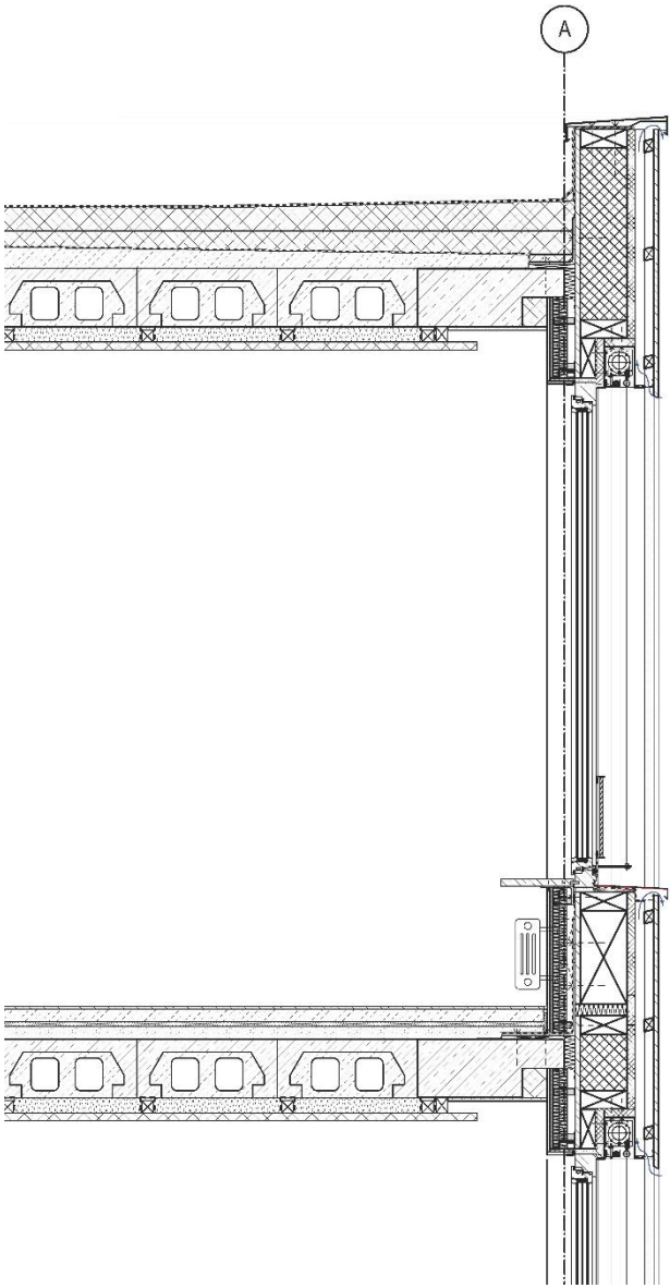
Fassadenschnitt Bestand und Wandmontage
