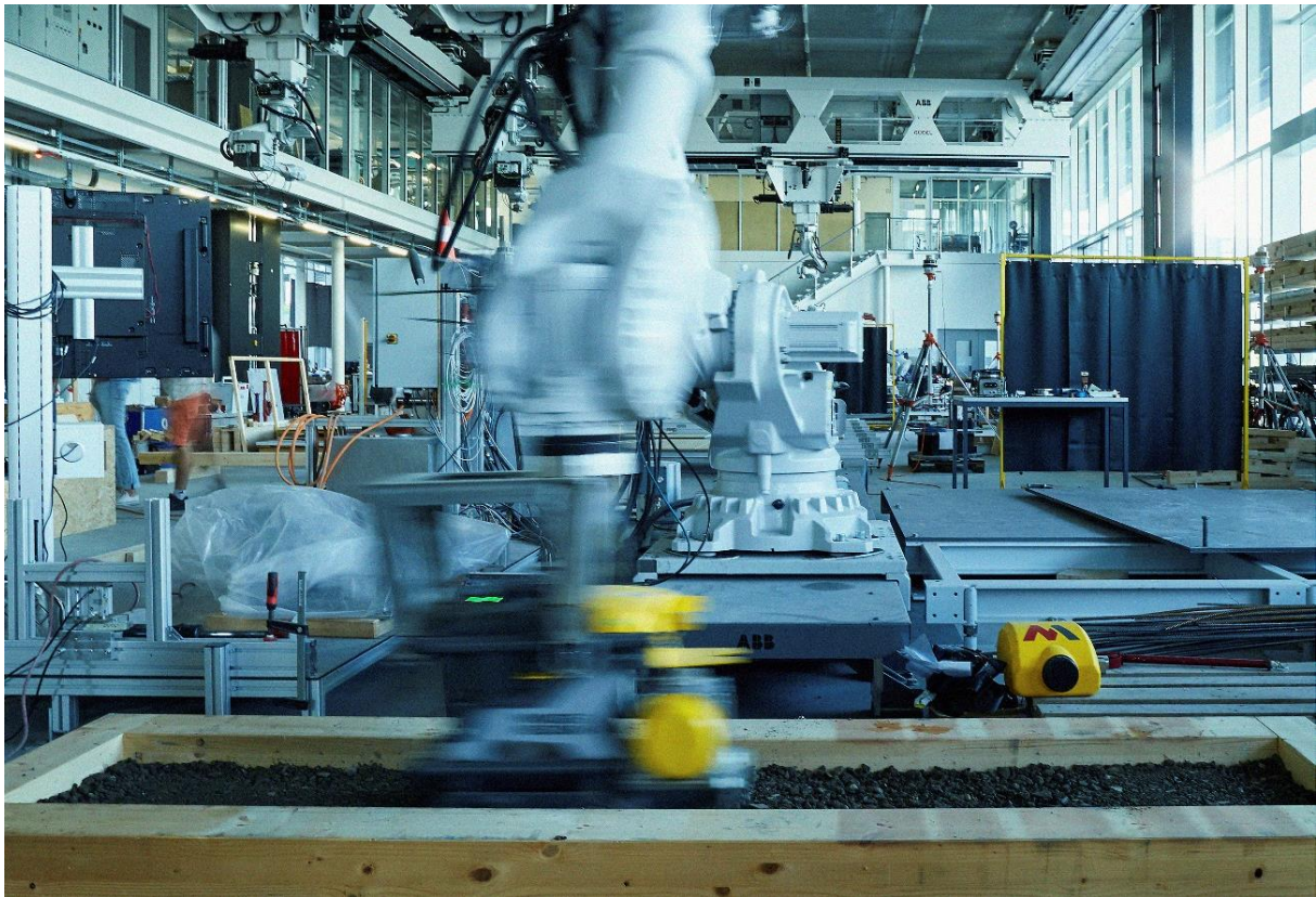
Abbildung 7: Versuch für die automatisierte Herstellung eines Holz-Lehm-Deckenelements; Foto © Ephraim Bieri
