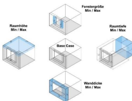
Abbildung 4: Jeweils ein Parameter der Grundvariante wurde schrittweise verändert
