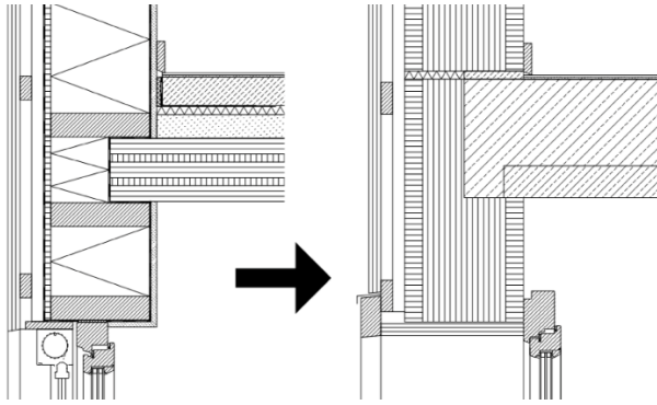
Abbildung 2: Schematische Darstellung des vereinfachten Wandaufbaus in Holz
