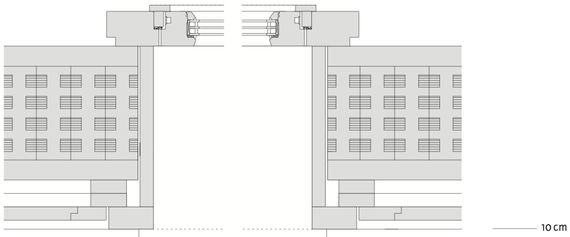
Abbildung 9: Ausführungsplanung für eins der drei Forschungshäuser für Bad Aibling. Architekt Florian Nagler hat hier Vollholzwandbauteile mit schmalen Schlitzen in den vertikalen Mittellagen verwendet. Einem Hohlkammerziegel ähnlich verringern die Lufteinschlüsse die Wärmeleitfähigkeit der Bauteile. (Florian Nagler Architekten)
