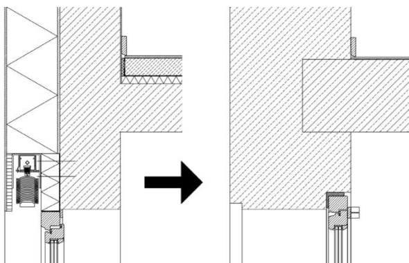
Abbildung 1: Schematische Darstellung des vereinfachten Wandaufbaus in Beton
