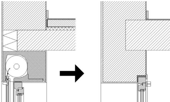
Abbildung 3: Schematische Darstellung des vereinfachten Wandaufbaus in Mauerwerk
