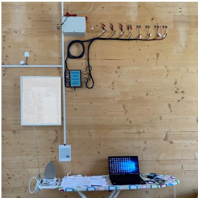
Abbildung 11: Bauteilmessung im Holzmassivhaus in Bad Aibling; Foto: TUM
