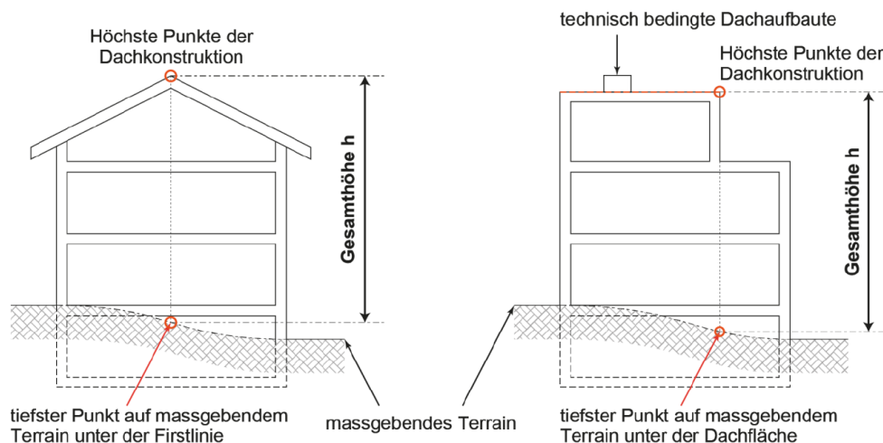
Abbildung 2: Messweise der Gesamthöhe
