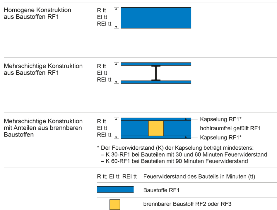
Abbildung 5: Anforderung an Aufbau, Materialisierung und Schichtigkeit von feuerwiderstandsfähigen Bauteilen, die Konstruktionen de RF1 entsprechen (Quelle VKF)
