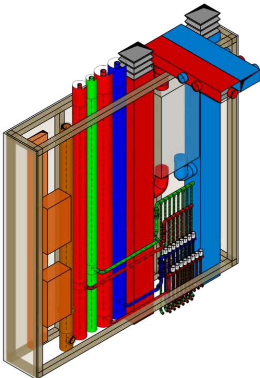
Abbildung 4: Typ L: Heizung, Lüftung, Sanitär, Elektro / Multimedia integriert
