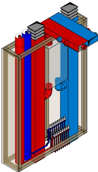
Abbildung 2: Typ S, Heizung und Lüftung integriert
