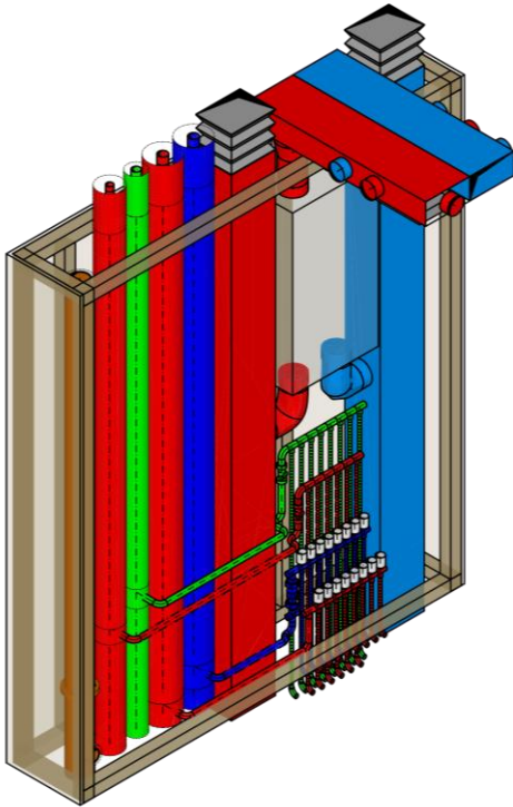
Abbildung 3: Typ M, Heizung, Lüftung und Sanitär integriert
